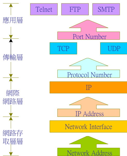
圖 1-17 TCP/IP 各層次的定址名稱
