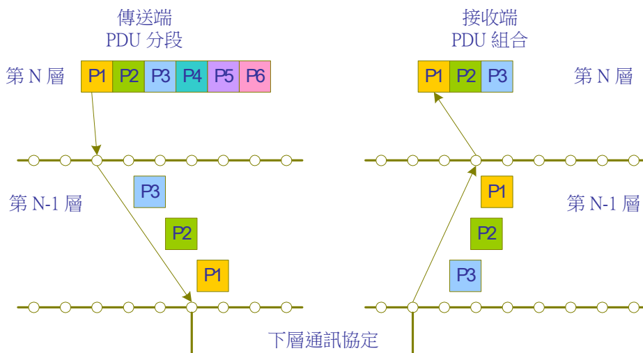
圖 1-7 協定資料單元之分段與組合
