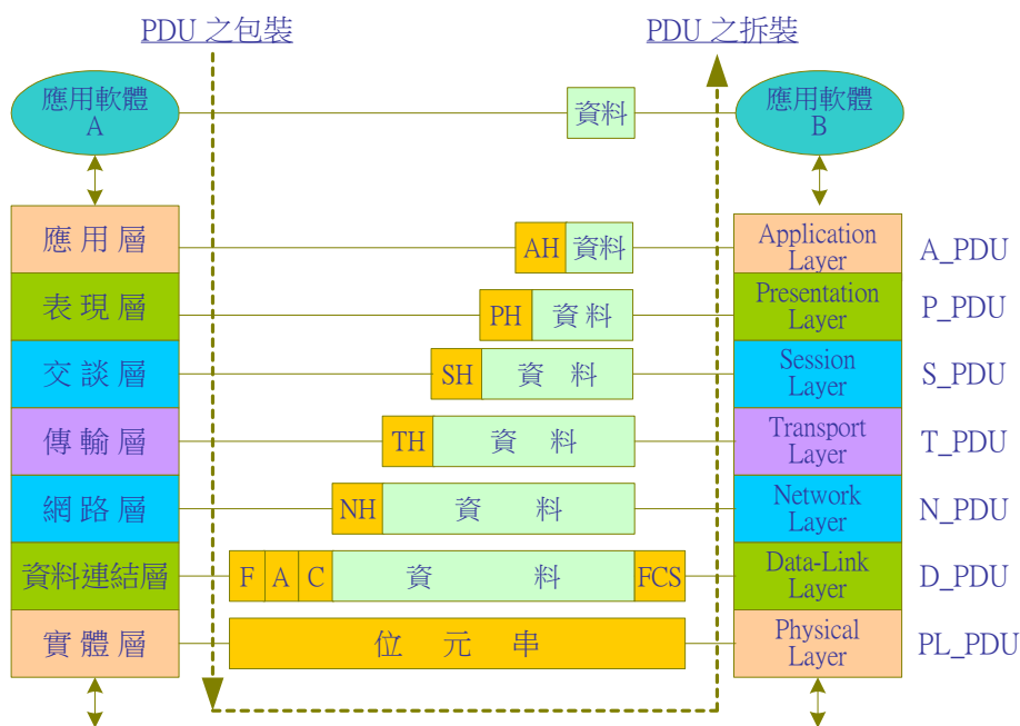
圖 1-6 協定資料單元之包裝與拆裝
