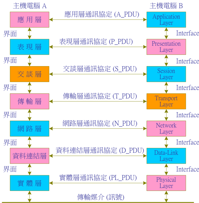
圖 1-10 OSI 參考模式
