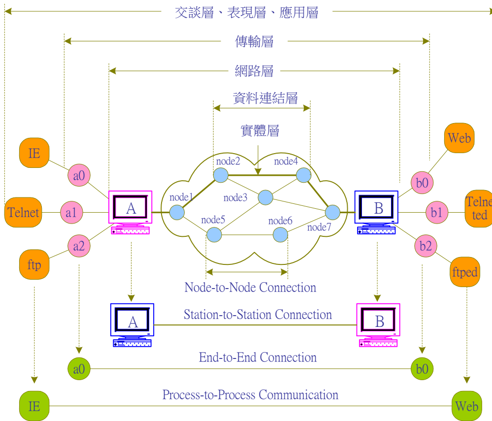
圖 1-12 TCP/IP 網路各層次連結功能
