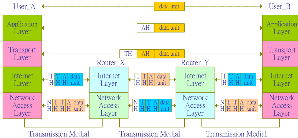
圖 1-15 TCP/IP 之協定資料單元的包裝
