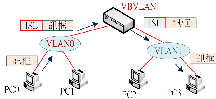
(B) 虛擬區域網路圖
