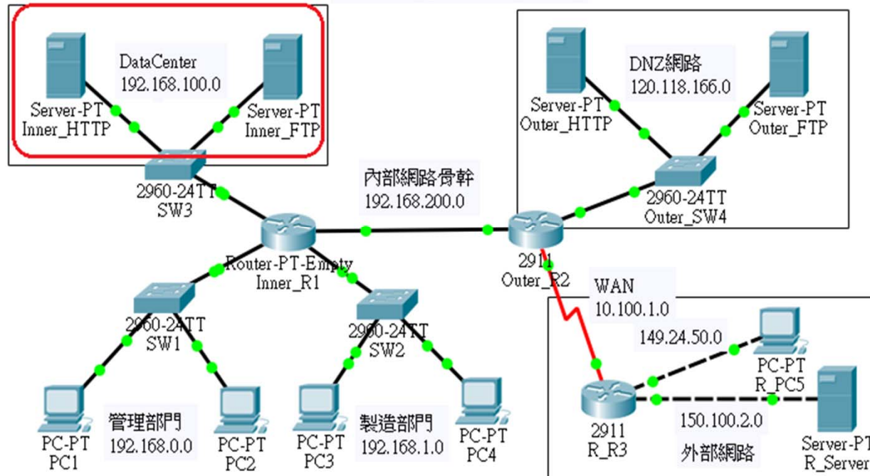
DNZ防火牆_內部伺服主機設定
