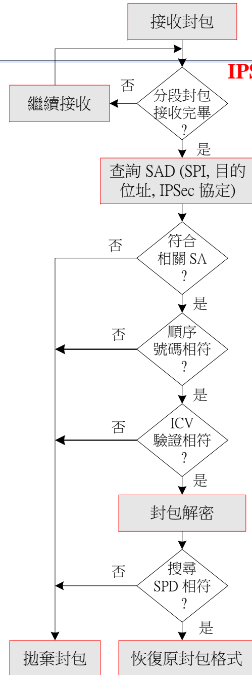
(b) 接收 IPSec ESP 運作程序
