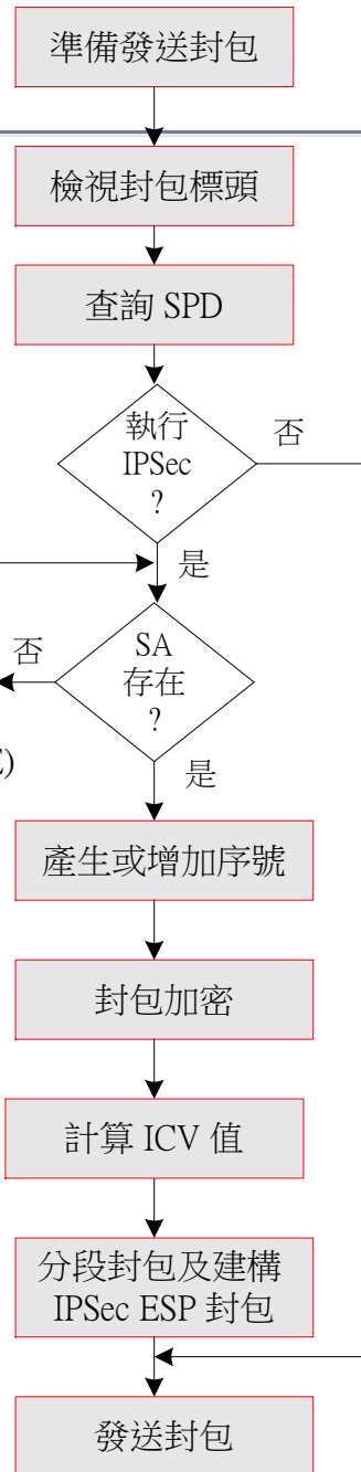
(a) 送出 IPSec ESP 運作程序
